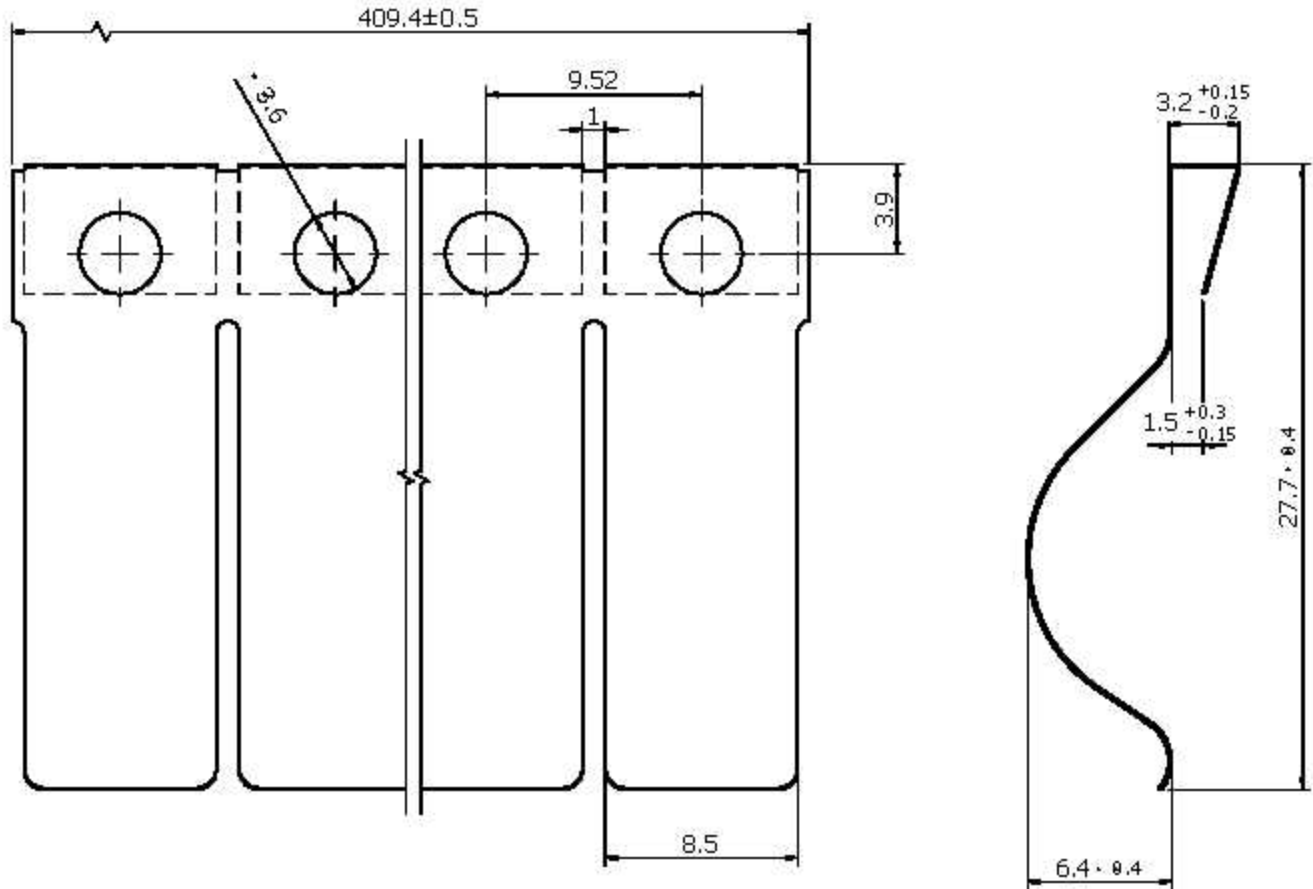
FEA656 FINGER GASKET 43 PINS (BeCu1720, 0.12t)
